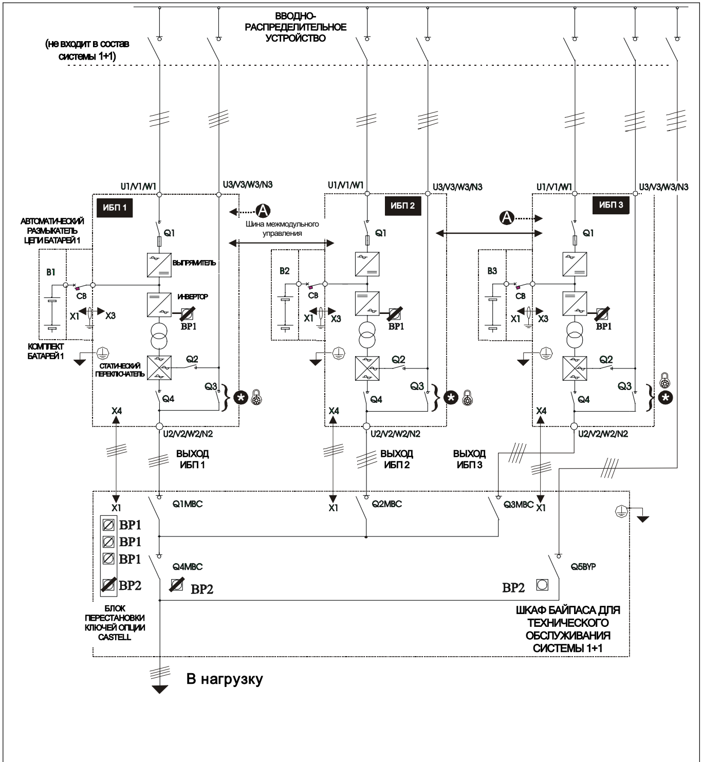
Рисунок 4.5 Пример конфигурации системы из трех ИБП, соединенных параллельно, со шкафом внешнего технического байпаса
