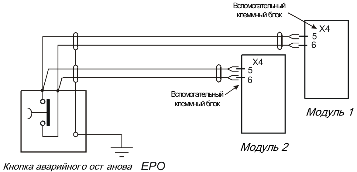
Рисунок 4.3 Схема соединения кнопки аварийного останова для двух модулей.
