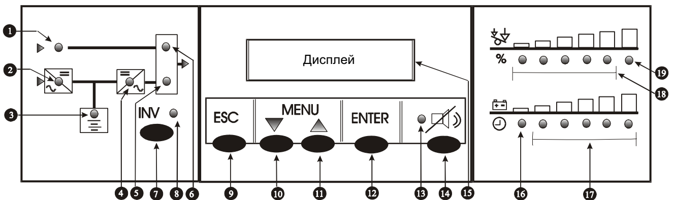
Рисунок 8-2 Панель управления оператором – расположение элементов
