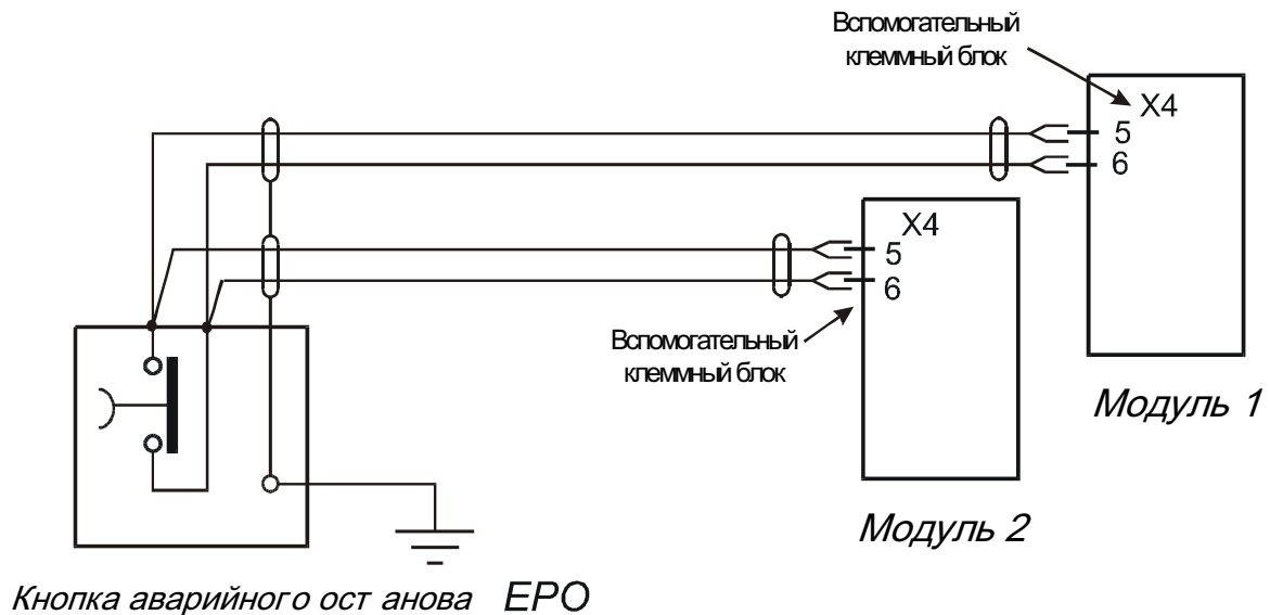
Рисунок 10-1 Подключение кнопки аварийного останова (ЕРО).
