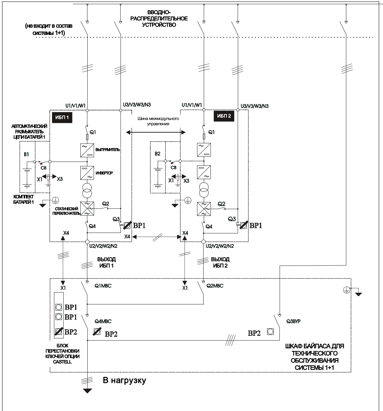
Рисунок 4.4 Схема-пример конфигурации параллельного соединения двух ИБП для избыточности со шкафом внешнего технического байпаса.
