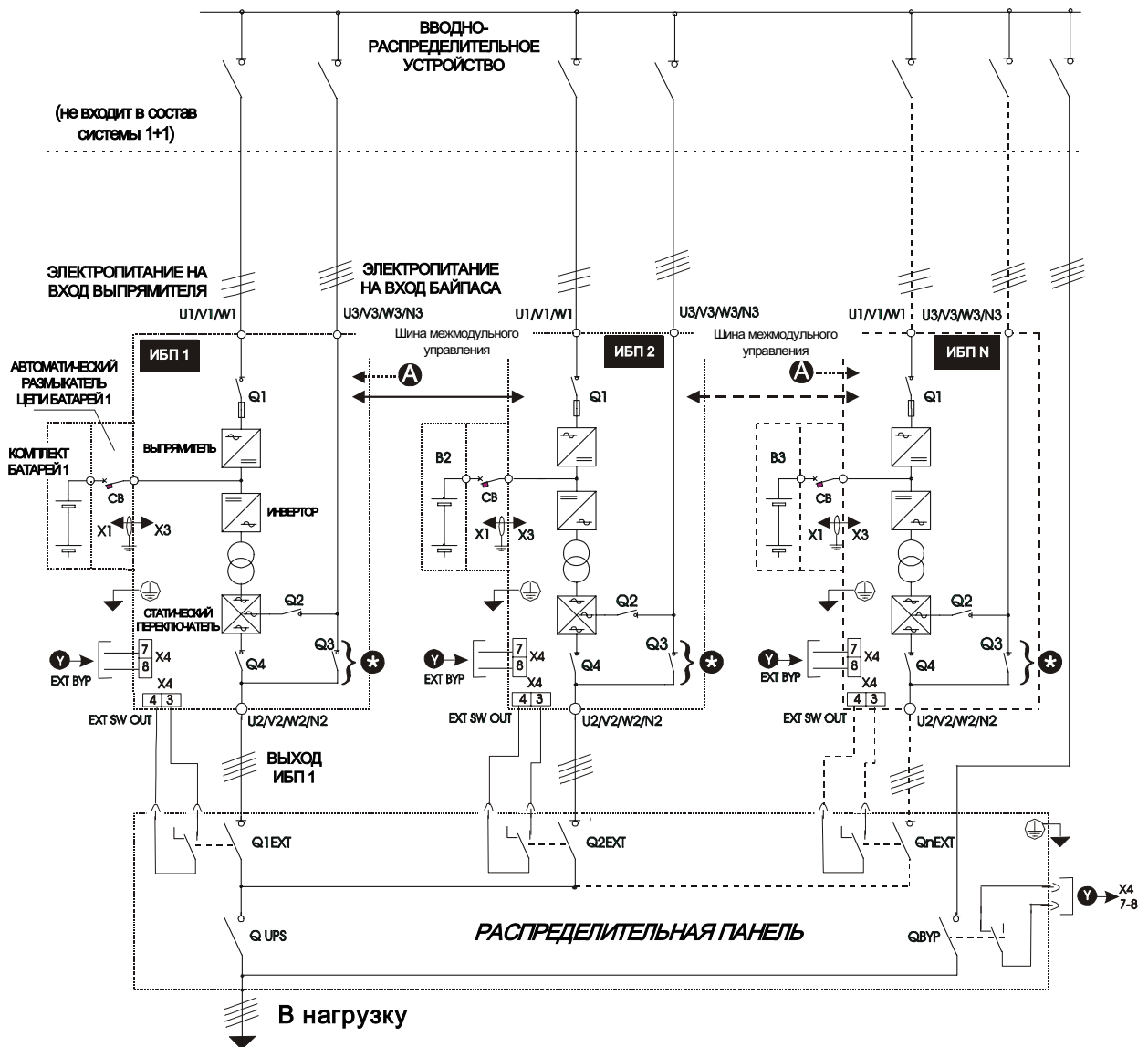
Рисунок 4.1 Структурная схема параллельной системы 1+N.
