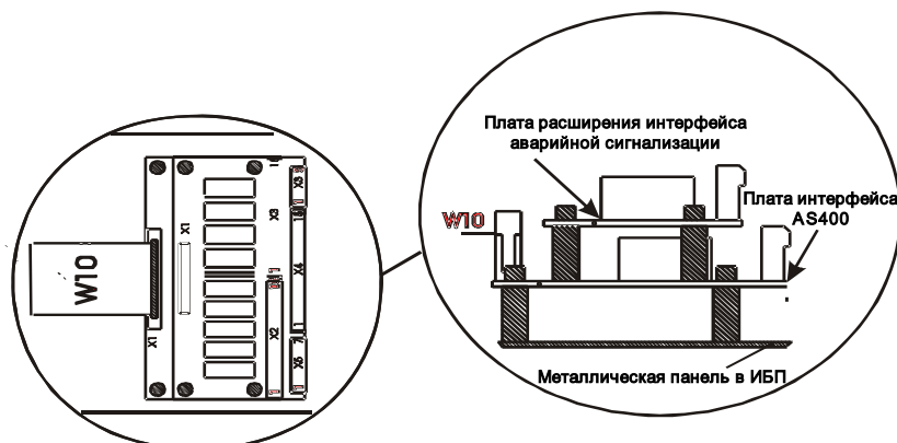
Рисунок 12.1 – Платы Интерфейса аварийных сигналов – детали установки
