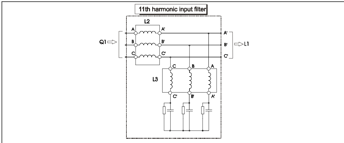
Рисунок 12-4 – Схема опционального входного фильтра гармоник
