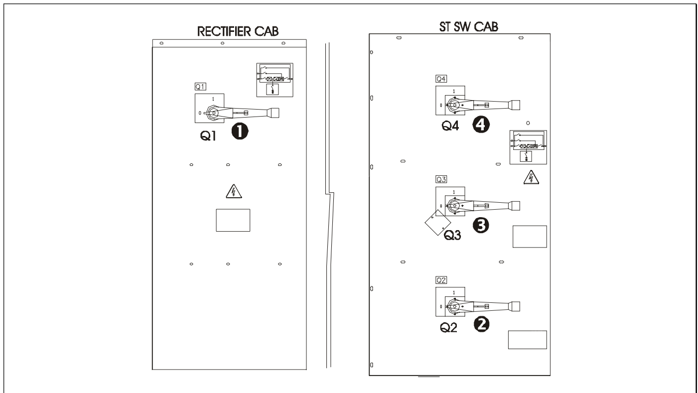
Рисунок 9-1 Расположение силовых выключателей
