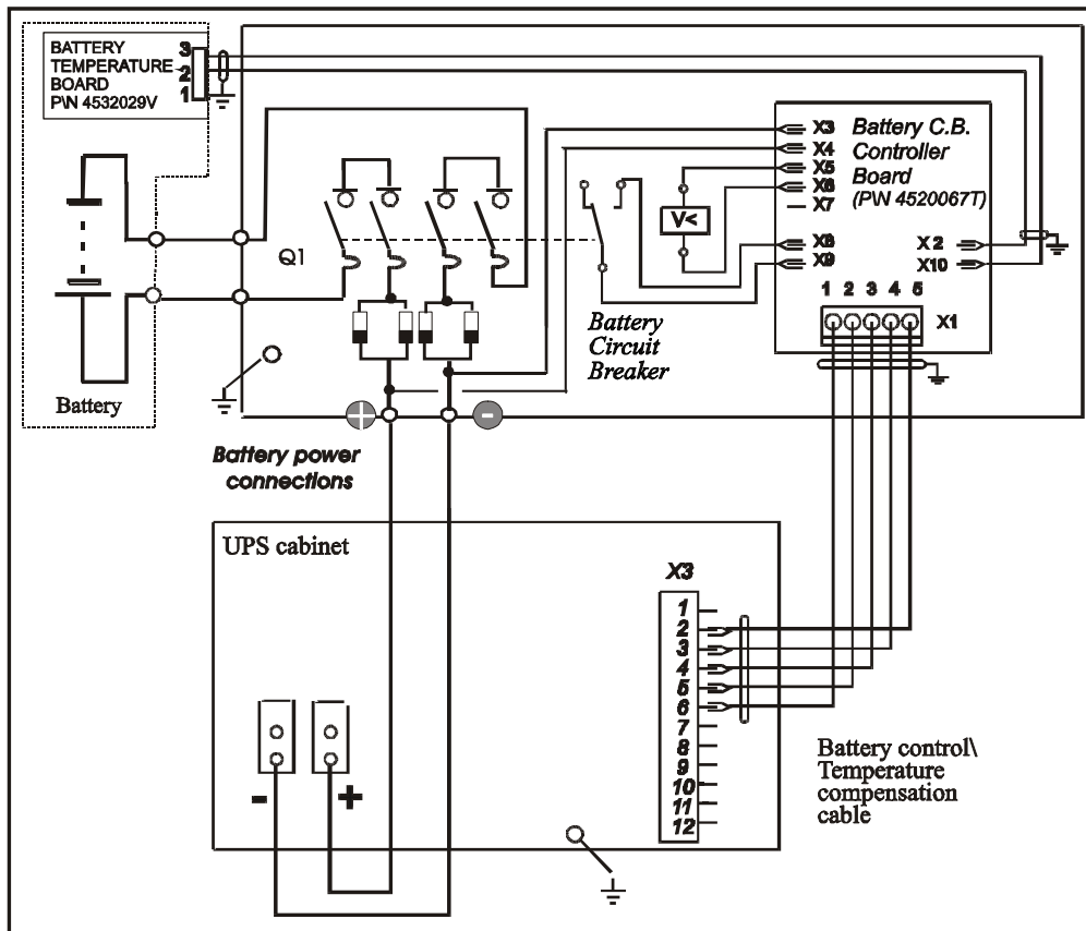
Рисунок 2.2 Батарейные соединения
