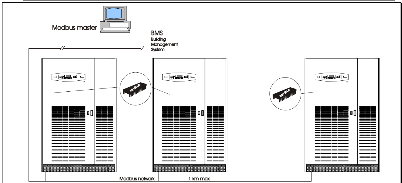
Рисунок 12-6 – Соединения для совместимости с протоколом Modbus
