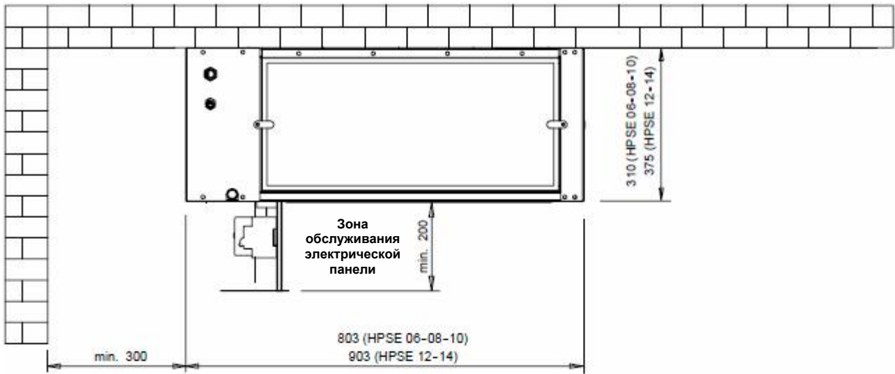
Рис. 14 – Монтаж модуля испарителя к потолку HPSE 06 – 08 – 10 – 12 – 14 (версия без фрикулинга)
