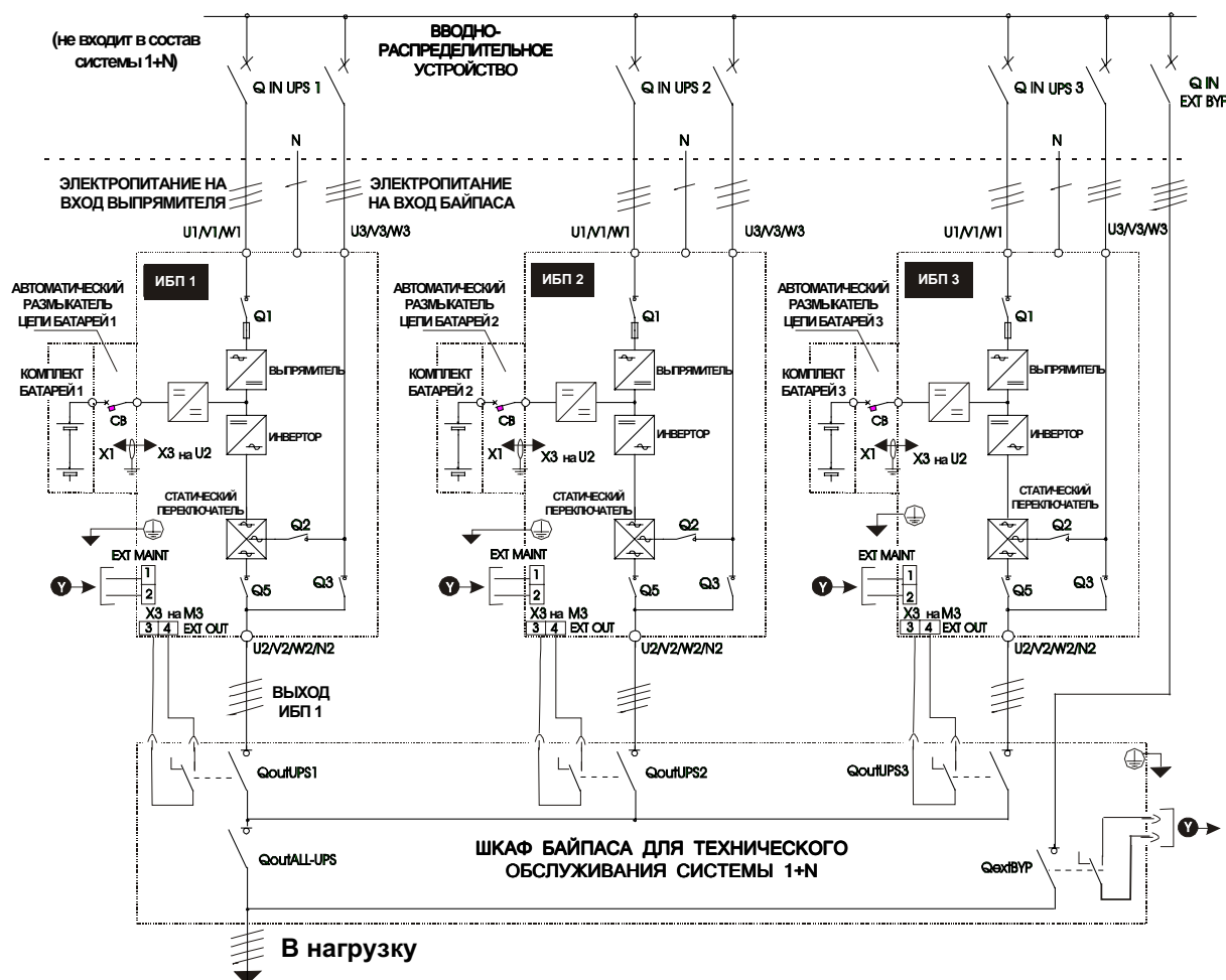
Рисунок 64 - Многомодульная система ИБП конфигурации 1+N с внешним выключателем байпаса для обслуживания
