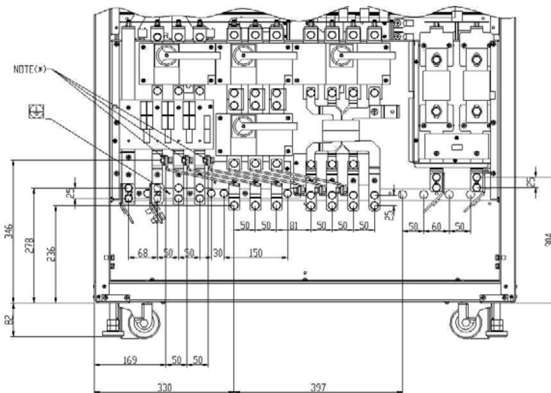
Рисунок 56 - ИБП NXa 140-200 кВА, силовое подключение
