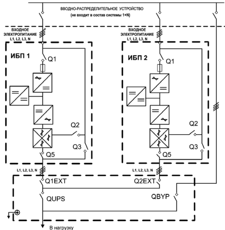
Рисунок 66 - Пример схемы подключения параллельной системы конфигурации '1+1' с внешним шкафом байпаса для технического обслуживания и подачи электропитания от одного общего источника
