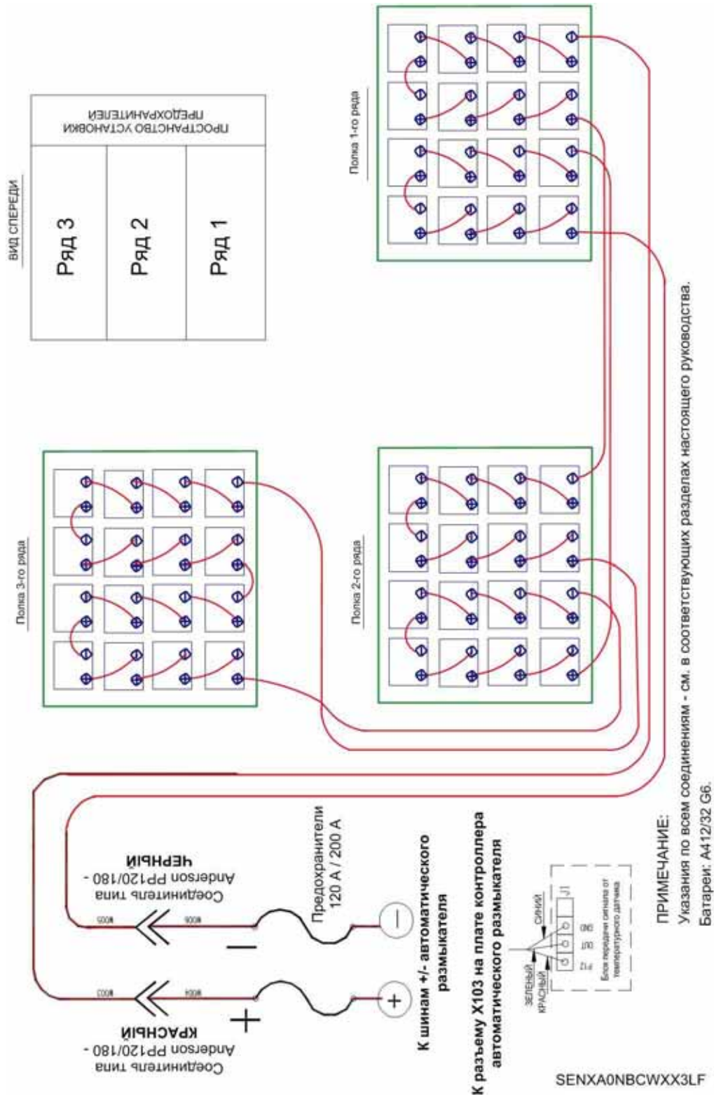
Рисунок 18 – Широкий шкаф батарей (3 полки) с предохранителями
