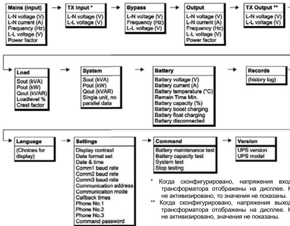
Рисунок 69 – Система меню
