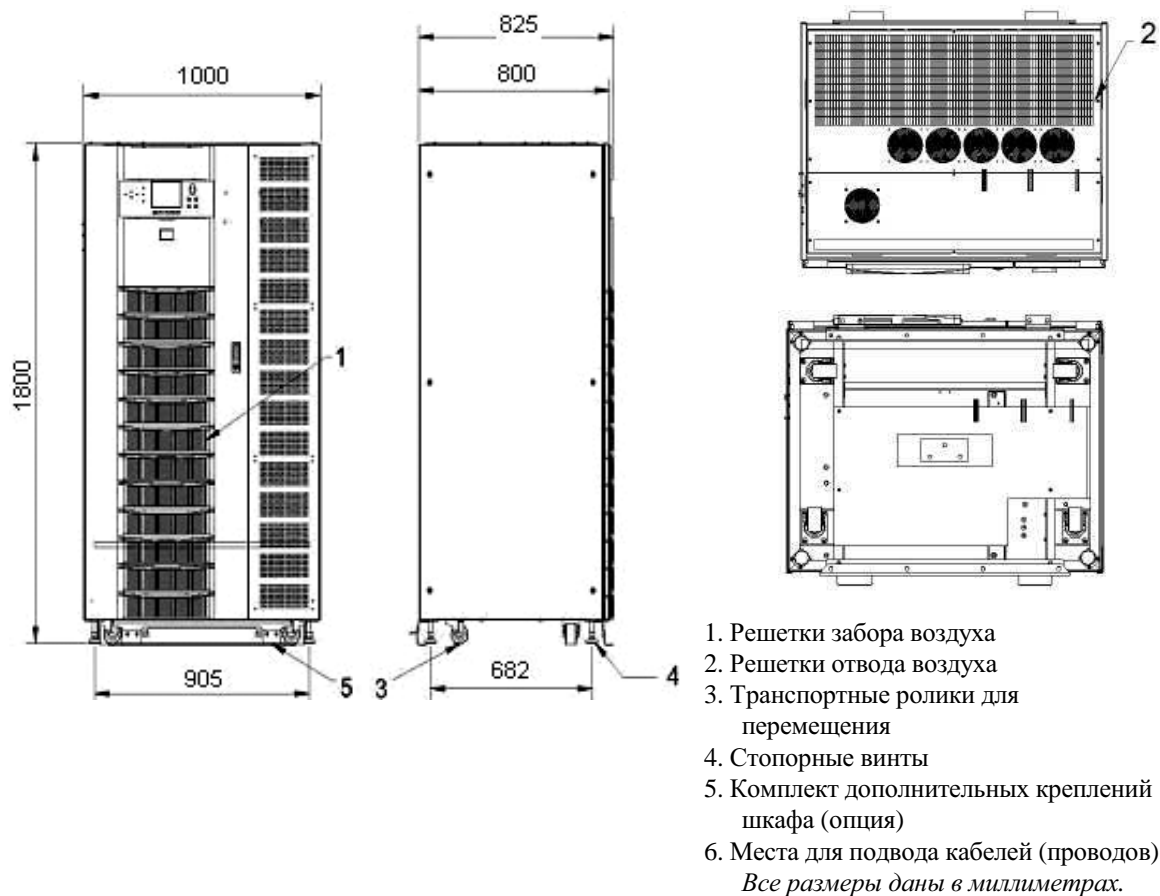
Рисунок 53 - ИБП NXa 140-200 кВА, основные размеры
